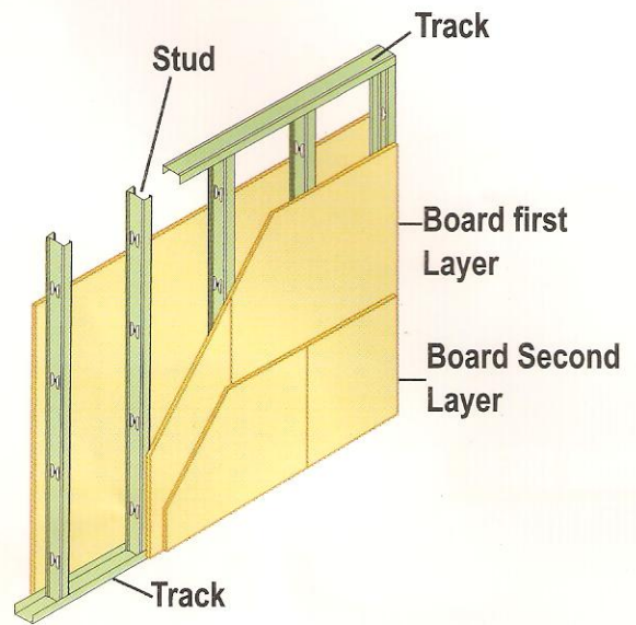
DOUBLE LAYER
